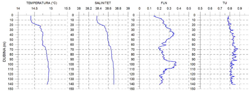
Vertikalni profili temperature, saliniteta, FLN i TU izmjerenih 02.03.2015. na postaji M150 (BIOTA).
