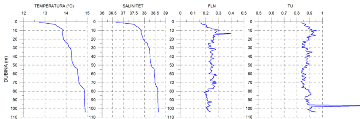
Vertikalni profili temperature, saliniteta, FLN i TU izmjerenih 28.02.2015. na postaji P100 (BIOTA).
