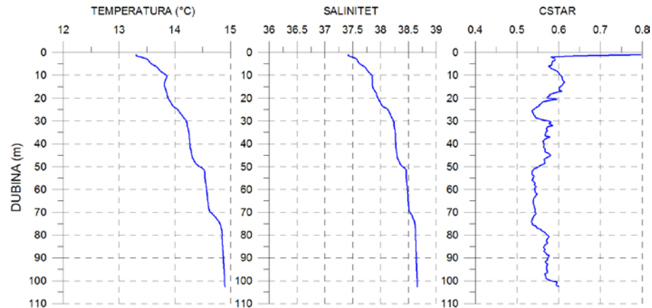
Vertikalni profili temperature, saliniteta i CSTAR izmjerenih 28.02.2015. na postaji P100 (BIOTA).
