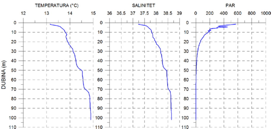
Vertikalni profili temperature, saliniteta i PAR izmjerenih 28.02.2015. na postaji P100 (BIOTA).
