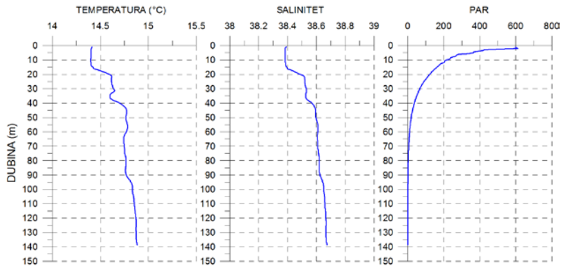
Vertikalni profili temperature, saliniteta i PAR izmjerenih 02.03.2015. na postaji M150 (BIOTA).
