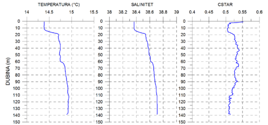
Vertikalni profili temperature, saliniteta i CSTAR izmjerenih 02.03.2015. na postaji M150 (BIOTA).
